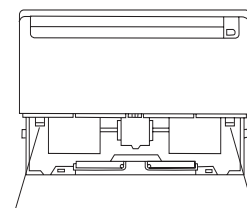
Abflussschlauch (links) Abflussschlauch (rechts)
